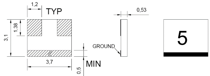
FAC0605 2W(Al 2 O 3 ) 公差±0.1
