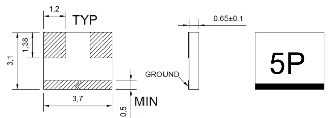
FAC0605P 5W(BeO) 公差±0.1
