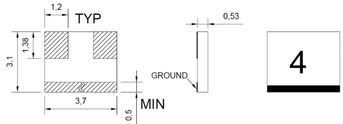
FAC0604 2W(Al 2 O 3 ) 公差±0.1
